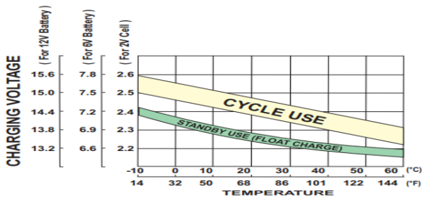
Quan hệ giữa Điện áp và Nhiệt độ
