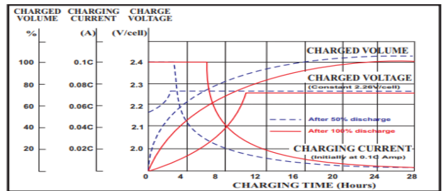
Đặc tính nạp điện
