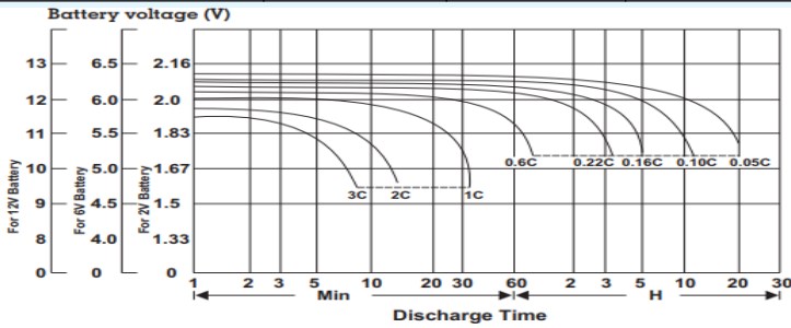
Đặc tính phóng điện
