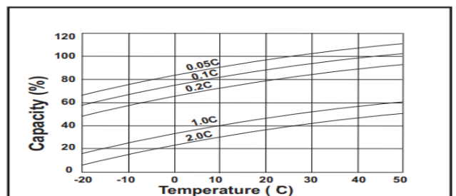
Mối quan hệ giữa nhiệt độ và dung lượng
