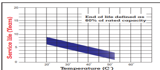
Ảnh hưởng của nhiệt độ đến tuổi thọ ắc quy sử dụng ở chế độ nạp nổi (Float)
