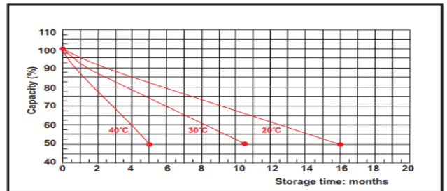
Đặc tính độ tự phóng
