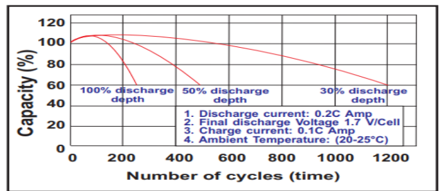
Mối quan hệ giữa độ sâu phóng và tuổi thọ
