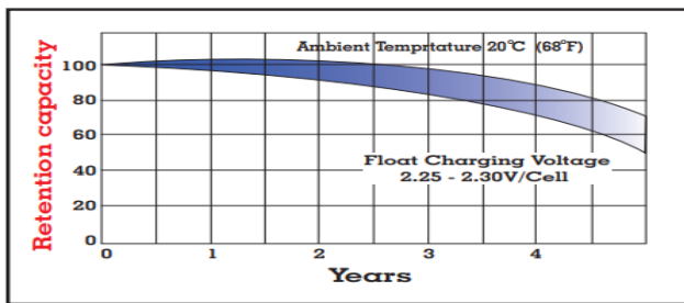
Tuổi thọ ắc quy ở chế độ nạp nổi (FLOAT)
