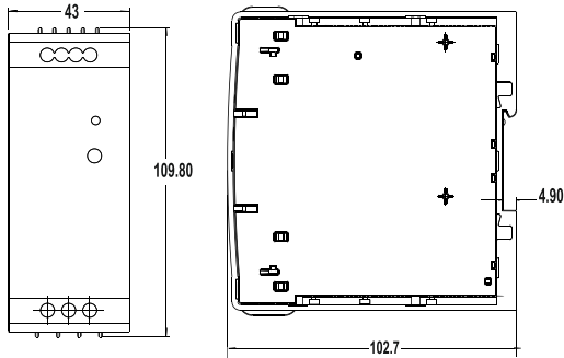
RPS60 / RPS120
