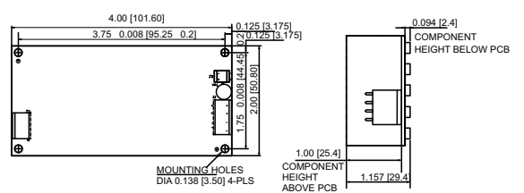
OPS2x4-150
