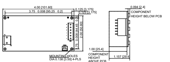
OPS2x4-200
