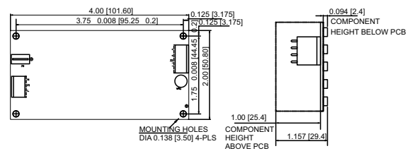
OPS2x4-150
